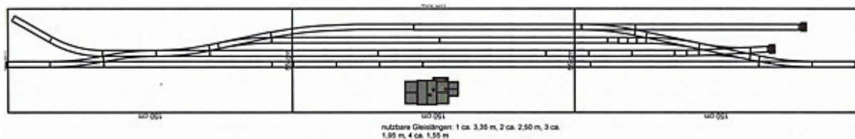
Schematischer Gleisplan
